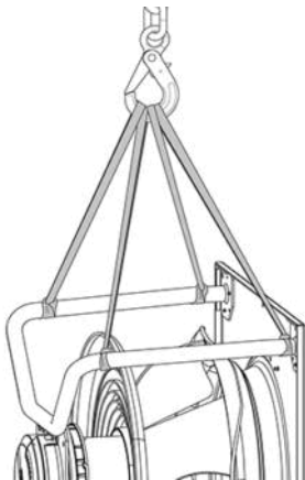
Abb. 1: Hebeskizze für den Transport des RadiPac
