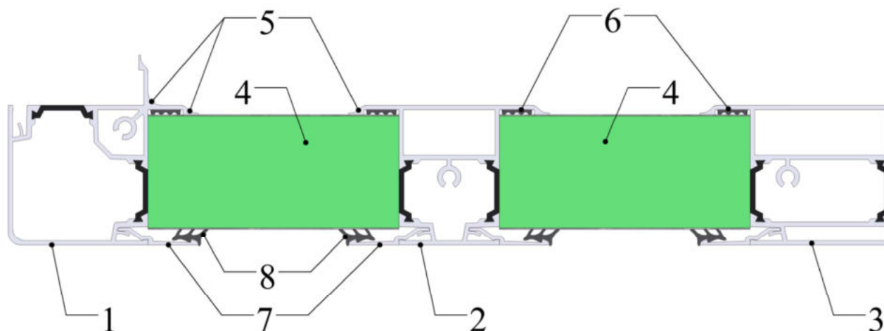
AmberAir Compact SD50+ Querschnitt
