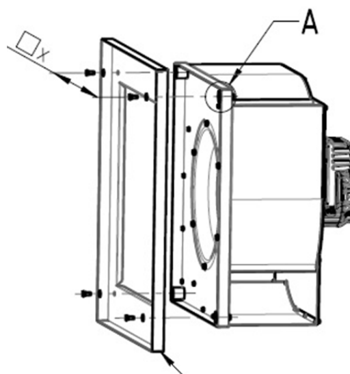
Kundenseitige Montagewand
