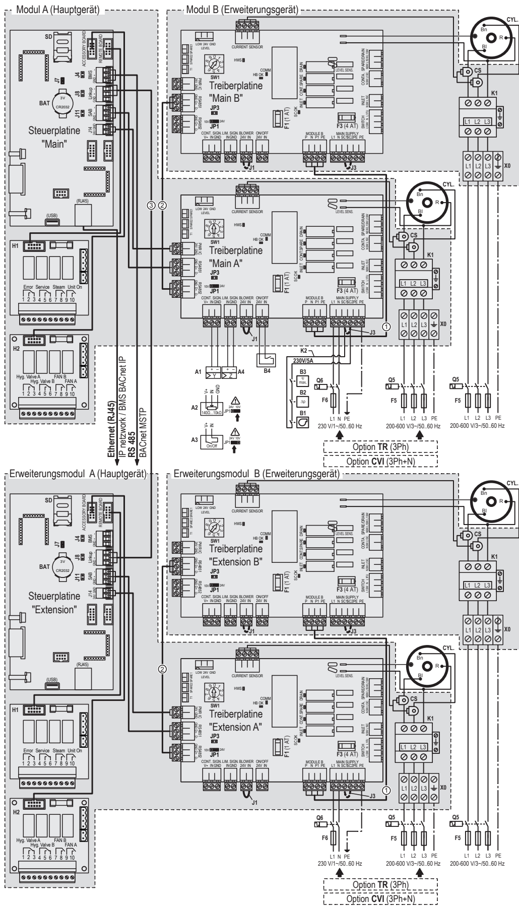
Abb. 28: Elektroschema Condair EL - Linkup-Systeme 100...160 kg/h
