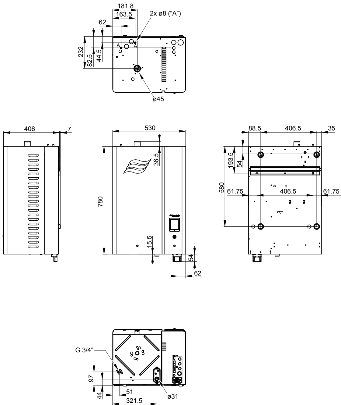
Abb. 30: Masszeichnung Condair EL 20 - 45 und EL 35 - 180, Gehäusegrösse "M" (Masse in mm)
