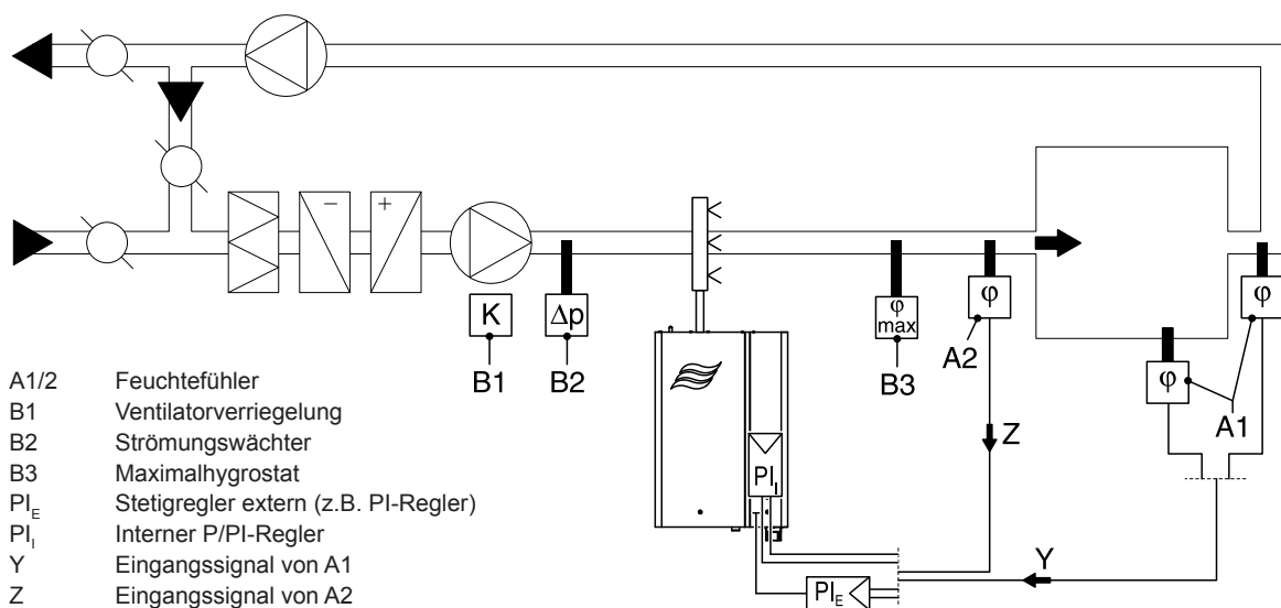
Abb. 23: System 2 – Raumfeuchteregelung mit stetiger Begrenzung der Zuluftfeuchte
