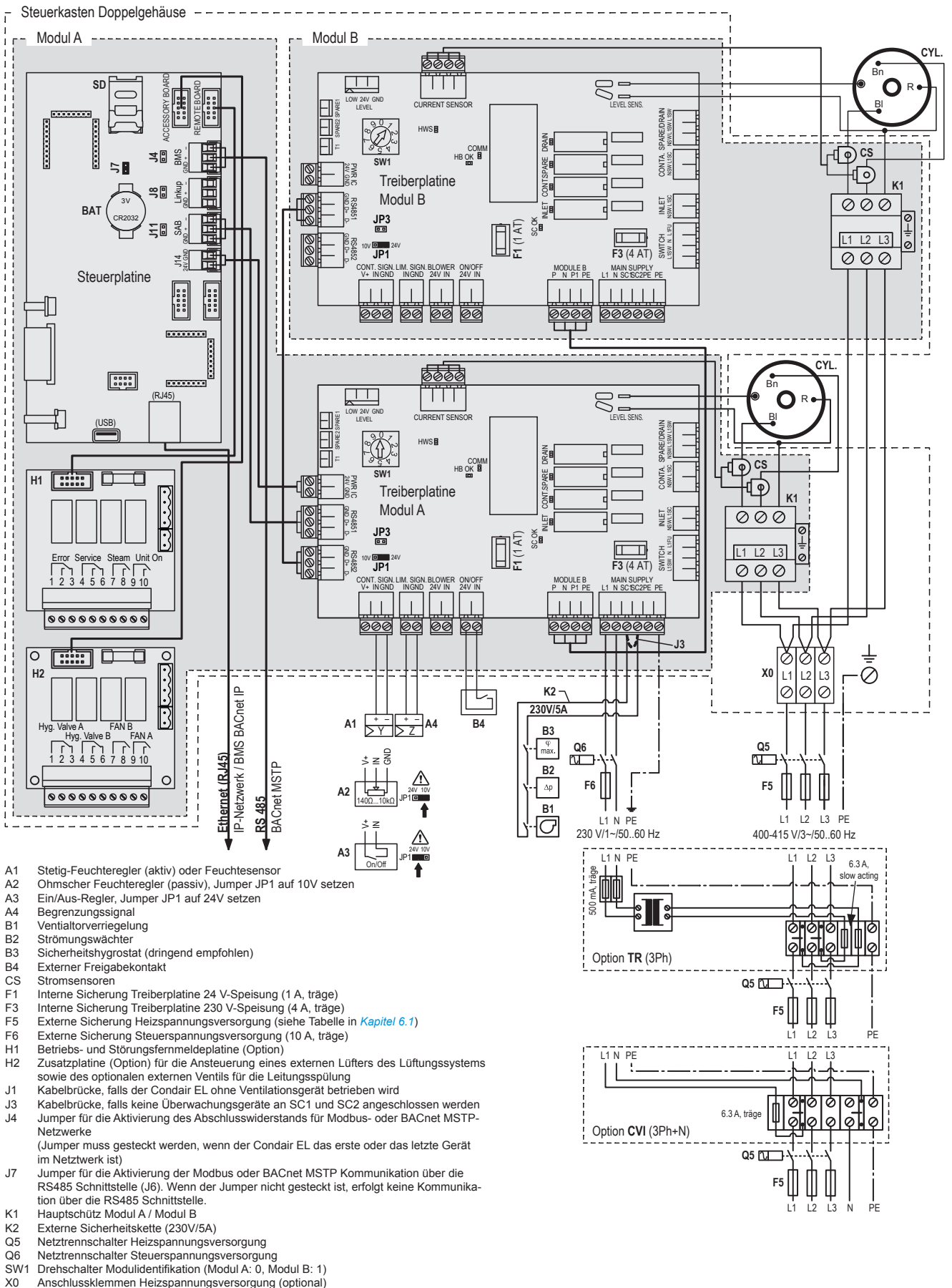
Abb. 26: Elektroschema Condair EL 50...90 - Einzelgeräte Gross ("L")
