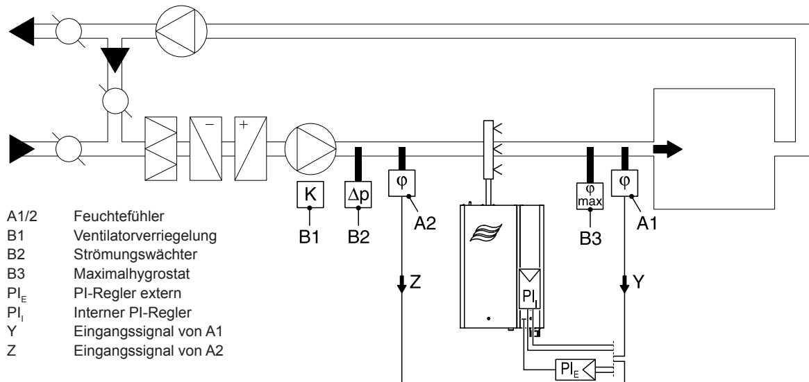
Abb. 24: System 3 – Zuluftfeuchteregelung mit stetiger Leistungsvorgabe
