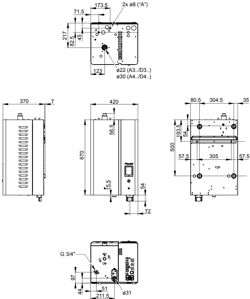
Abb. 29: Masszeichnung Condair EL 5 - 15, Gehäusegrösse "S" (Masse in mm)
