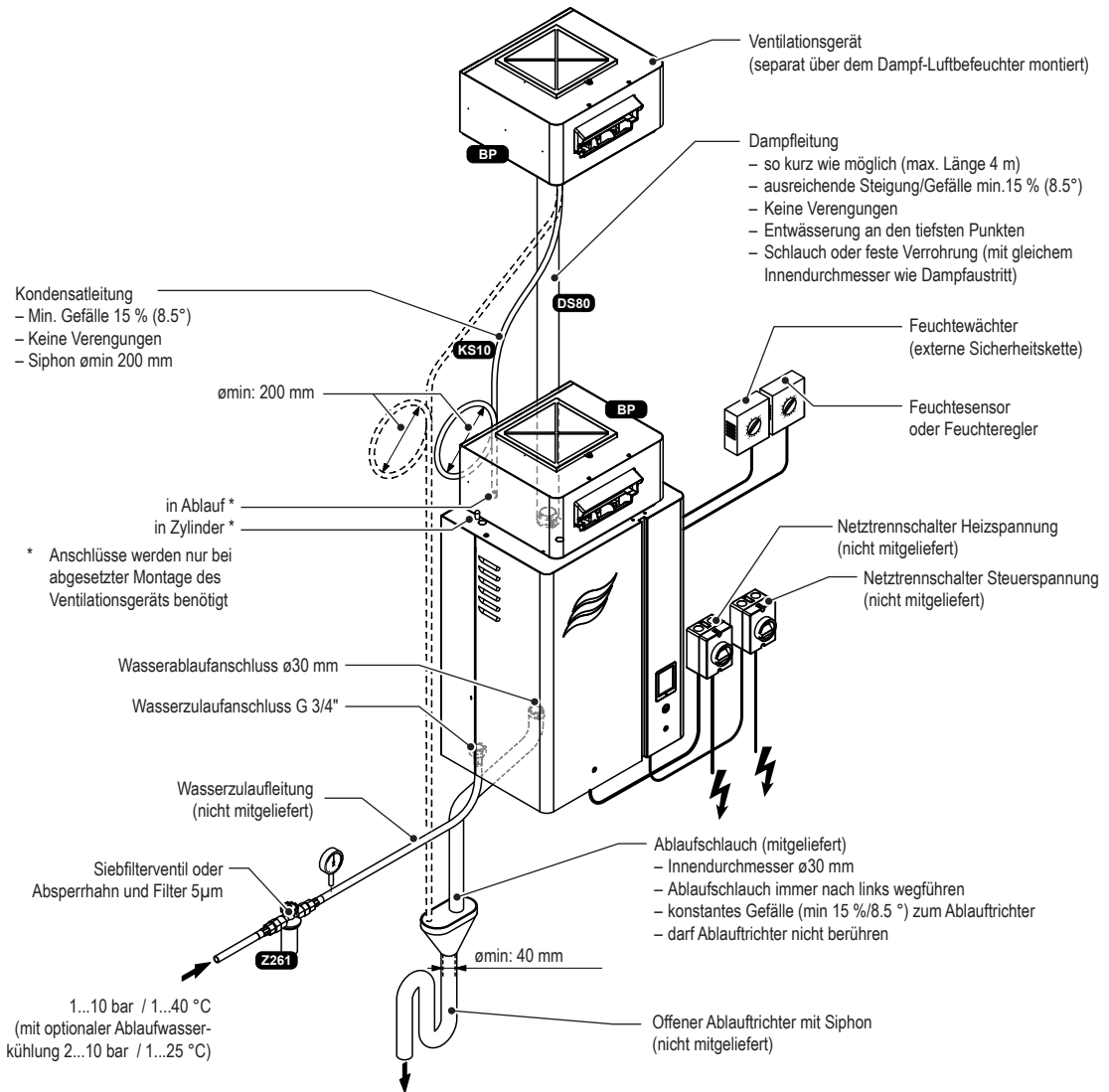
Abb. 8: Typische Installation für Direkt-Raumbefeuchtung
