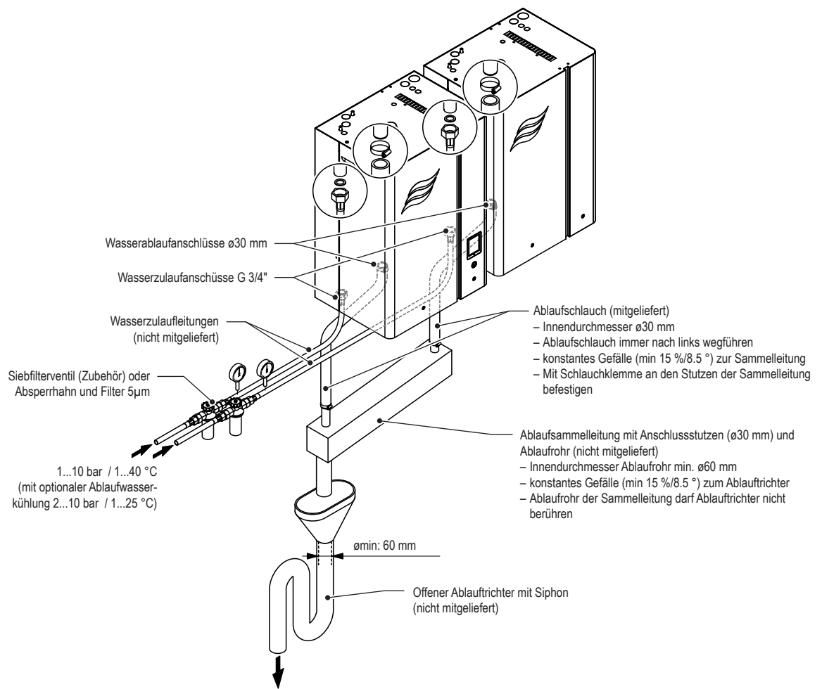
Abb. 21: Übersicht Wasserinstallation für Doppelgeräte Mittel ("M")
