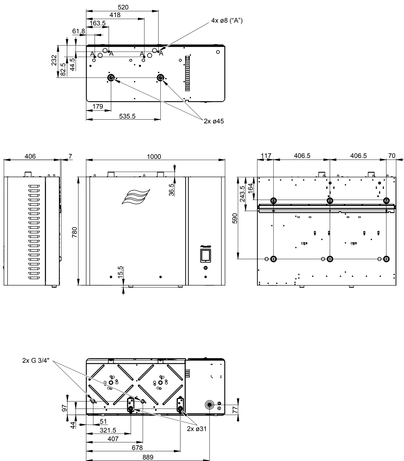
Abb. 31: Masszeichnung Condair EL 50 - 90, Gehäusegrösse "L" (Masse in mm)
