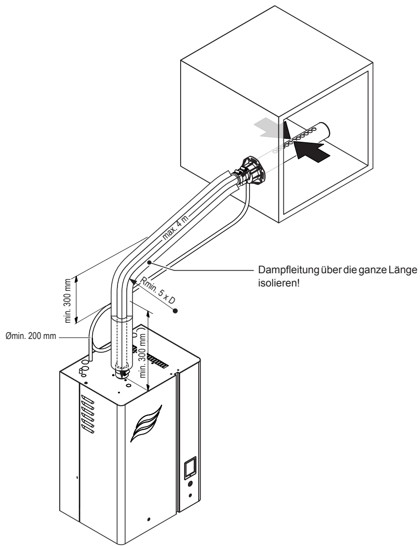
Abb. 17: Dampfleitung mit fester Verrohrung und Isolation
