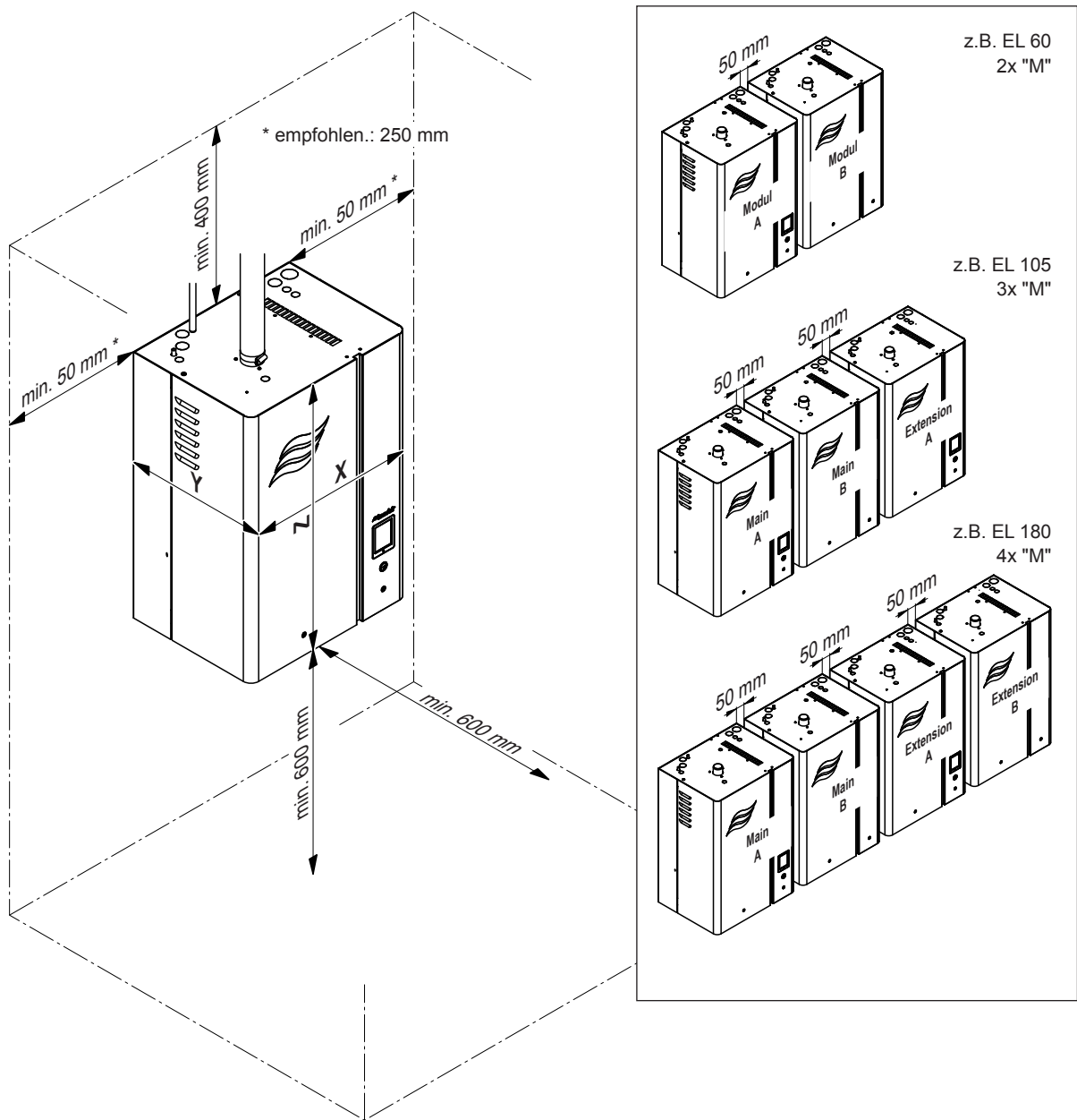
Abb. 9: Einzuhaltende Abstände
