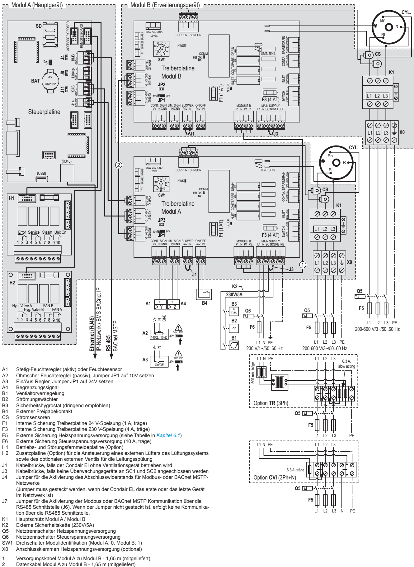
Abb. 27: Elektroschema Condair EL - Doppelgeräte (2 x "M") 40...80 kg/h
