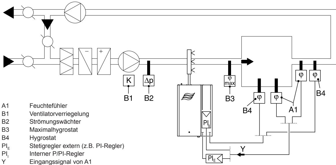
Abb. 22: System 1 – Raumfeuchteregelung
