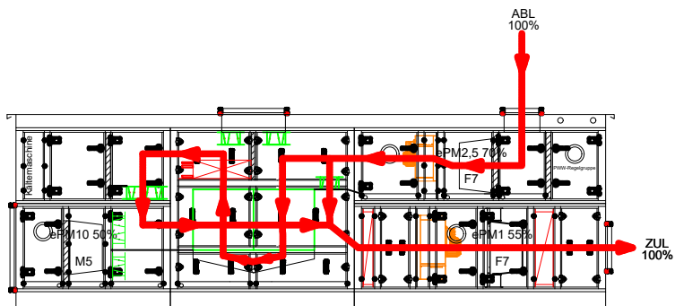
Ruhebetrieb 100% Umluftanteil
