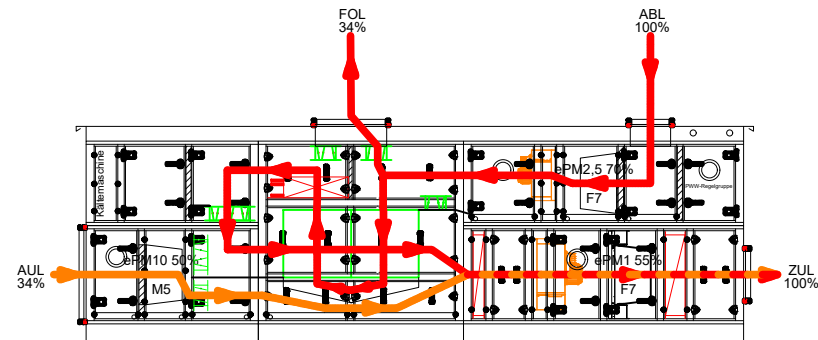
Badebetrieb 1/3 Außenluftanteil
