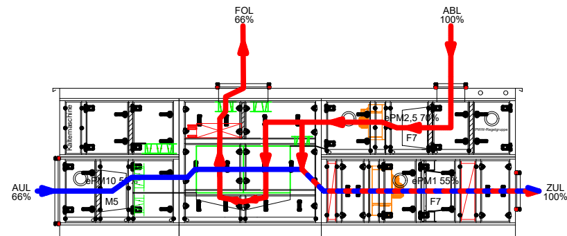
Winterbetrieb 2/3 Außenluftanteil
