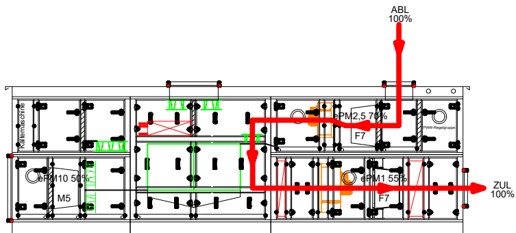
Aufheizbetrieb 100% Umluftanteil
