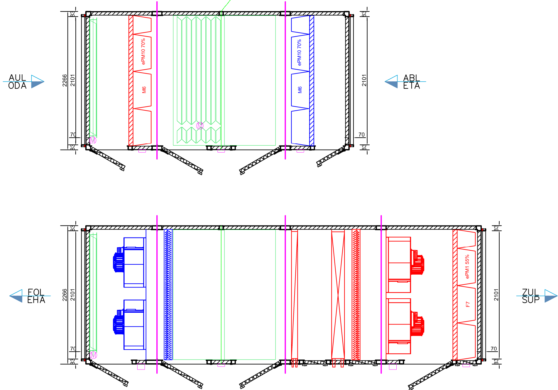
Teilung Deckel und Bodenschale
