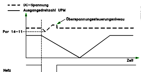
Abbildung 3.2: Rampenstopp, kurzer Netzausfall. Rampenstopp nach Rampe Auf zu Sollwert.
