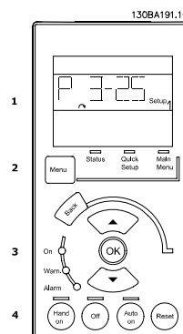
Abbildung 2.1: Numerische LCP Bedieneinheit LCP101
